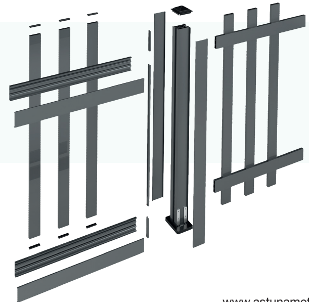
DERECE PROFİLİ DIŞ OUTER GRADE PROFILE
